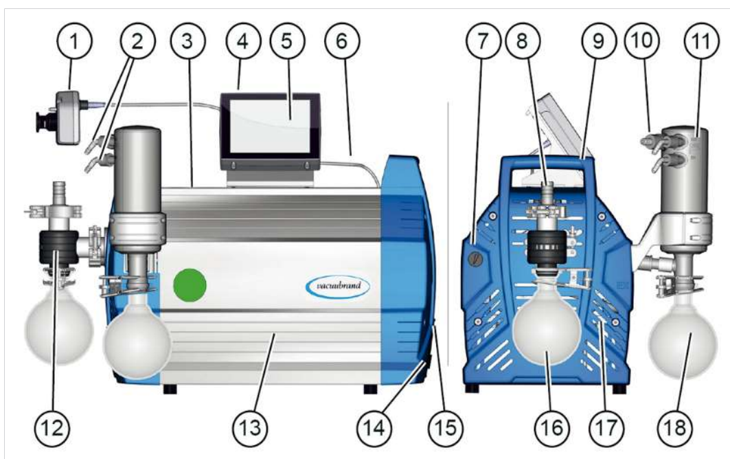
Aanzicht en principeopbouw PC 301x NT VARIO select
