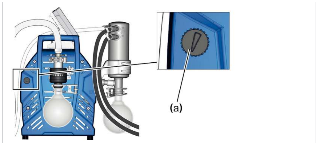
Positie gasballast-ventiel
