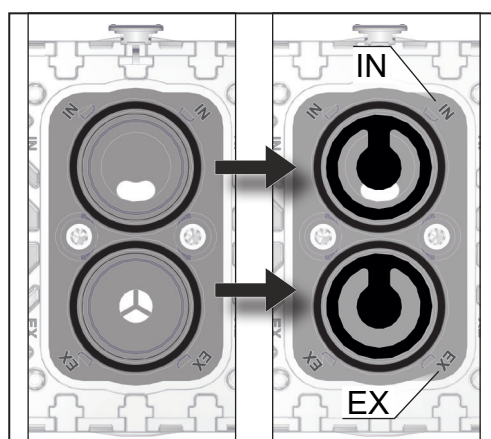
Vue de dessus détaillée : positionnement correct des clapets. IN = inlet (admission) EX = exhaust (ou outlet, échappement)
