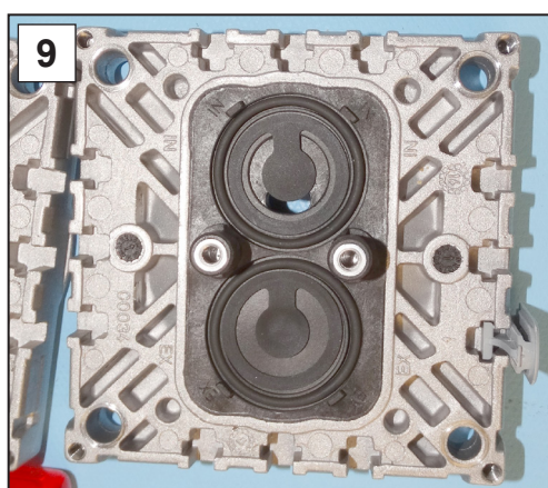
9. Posez les nouveaux clapets et orientez-les correctement.
