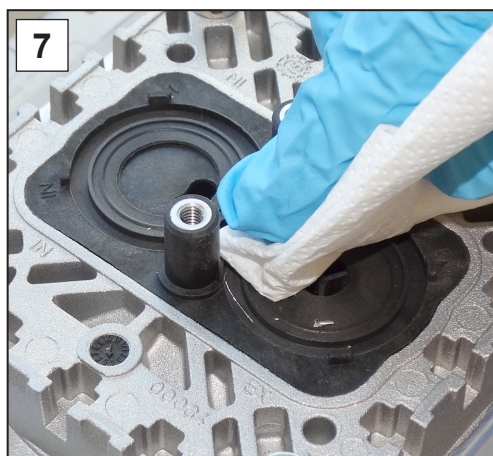
7. Nettoyez soigneusement toute surface encrassée.
