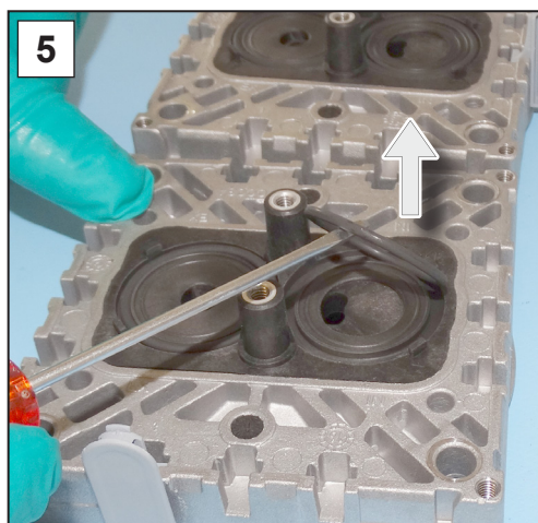
5. Retirez avec précaution les joints toriques et les clapets usagés.
