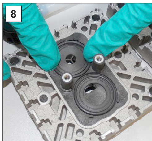
8. Posez des joints toriques neufs dans les rainures.
